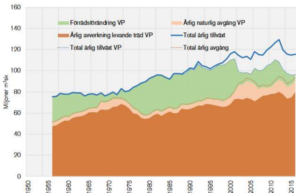
Bild 3. Historisk utveckling avseende tillväxt och avgång på total areal produktiv skogsmark och virkesproduktionsmark VP. Frivilliga avsättningar där ingen avverkning sker tillkom med den nya skogsvårdslagen 1993, och skall omfatta minst 5% av arealen och skall innehålla skyddsvärd skog. Riksskogstaxeringen Skogsdata 2020.
